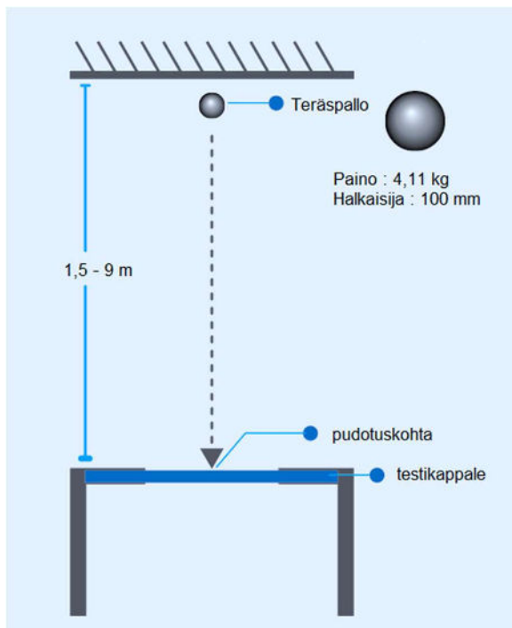
Kuva 8. Murtautumiskestävyys testaus teräskuulalla.
