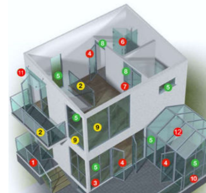
Kuva 5. Kuvasovellus asunnoille.
